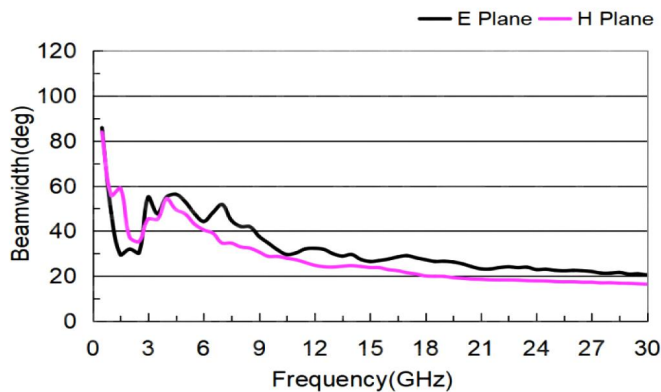
3dB Beamwidth
